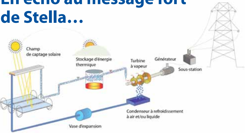
Principe de la production photothermique, Jean-Louis FULLSACK - Conférence Cerafrica - 27 01 2010
